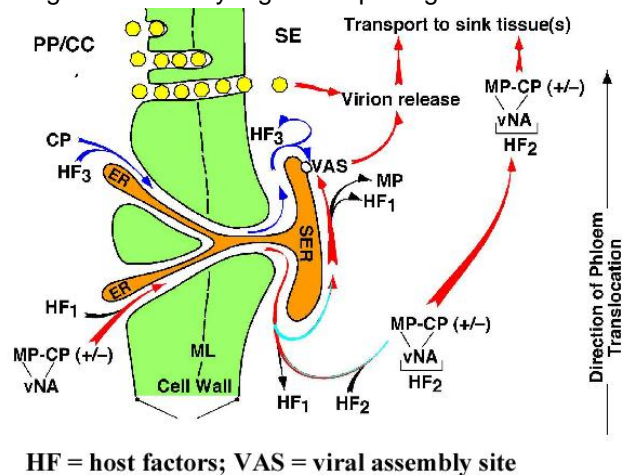
Gambar 1. Mekanisme Translokasi Virus di dalam Tubuh Tanaman
