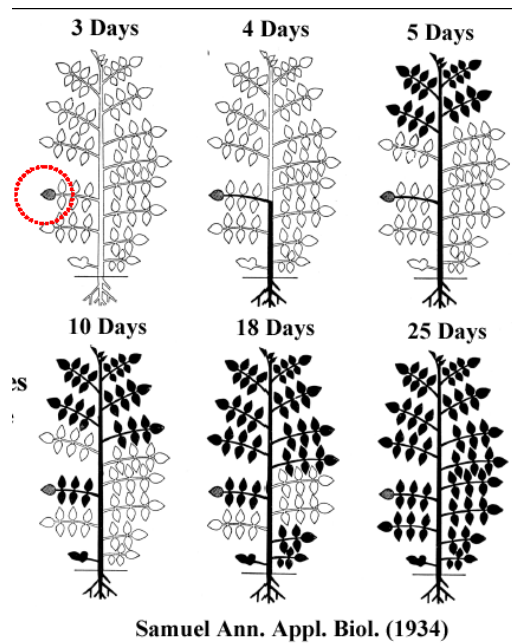
Gambar 2. Ilustrasi Proses Inveksi dan Penyebaran Virus di dalam Tubuh Tanaman
