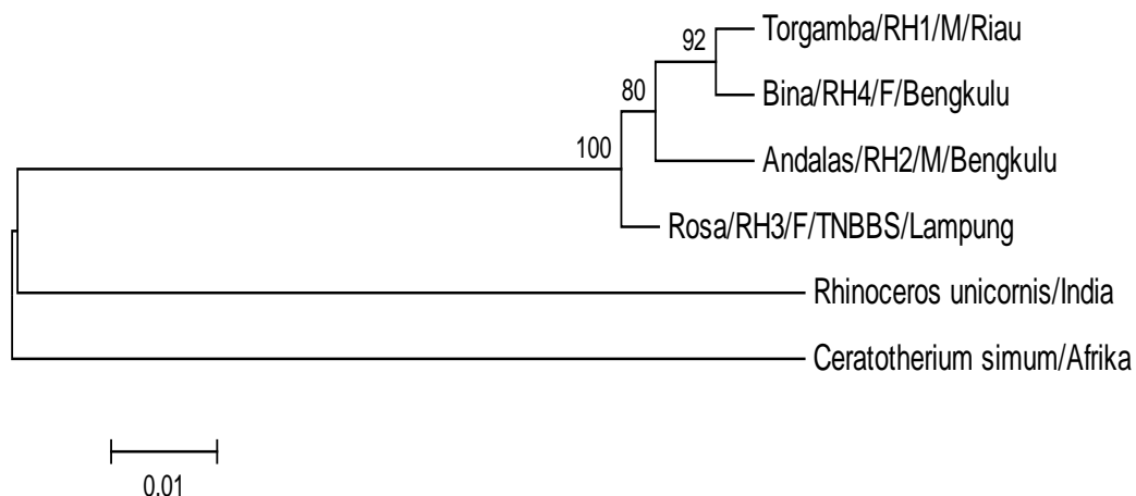
Gambar 1 Dendogram Neighbor-Joining dengan pengolahan bootstrap 1000 ulangan dari nukleotida daerah CO I parsial badak Sumatera, badak India dan badak putih Afrika (berukuran 711 nt)
