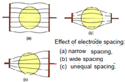
Gambar 14. Besar Elektroda yang Tepat
