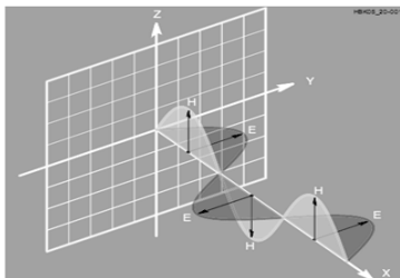
Gambar 15. Medan Listrik dan Magnet
