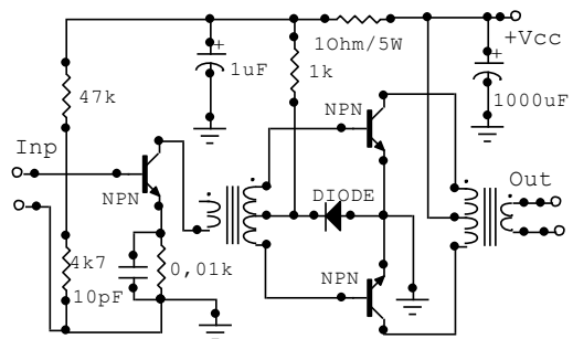
Gambar 21. Konverter
