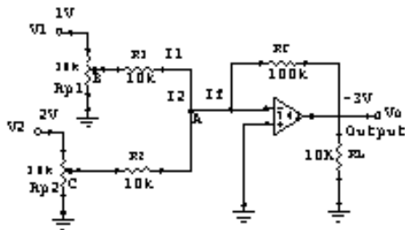
Gambar 20. Mixer Gelombang
