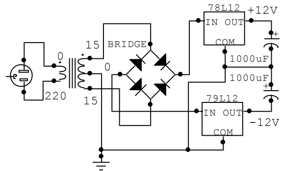
Gambar 22. Catu Daya
