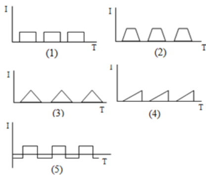
Gambar 11. Modifikasi Sinyal Impuls (J.F. Gabriel, 1996: 249)
