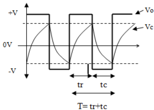
Gambar 18. Pengisian Pengosongan RC
