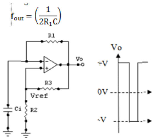
Gambar 17. Osilator Glb Kotak
