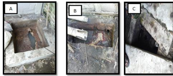
Gambar 1. Lokasi sampling pada tempat pembuangan limbah industri batik: A. Rumah Industri TN, B. Rumah Industri ER, C. Rumah Industri TG
