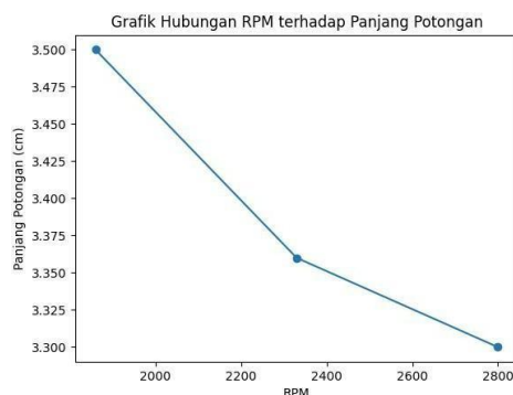
Gambar 2 Hasil Panjang Potongan terhadap RPM
