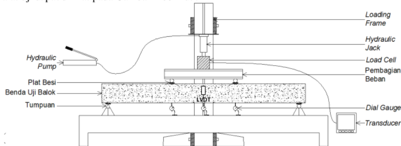
Gambar 2. Setting Up Alat Pengujian Balok
