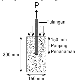
Gambar 1. Pengujian Pull Out .
