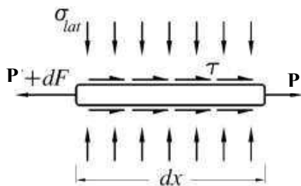
Gambar 2. Mekanisme Tegangan Lekatan pada Tulangan Tarik.
