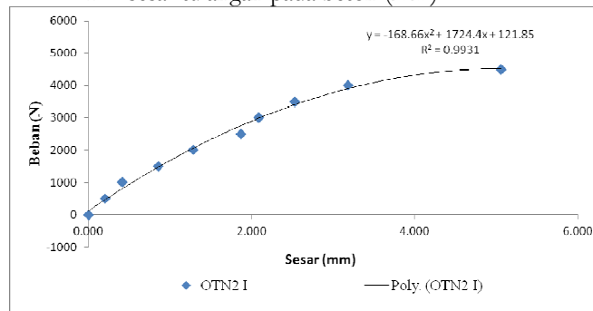
Gambar 6. Grafik Hubungan Beban-Sesar antara Beton dan Tulangan Bambu Ori Tanpa Nodia Takikan Bentuk V Jarak 20 mm.
