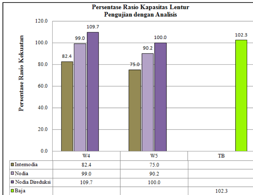
Gambar 8. Grafik Persentase Rasio Kapasitas Lentur Pengujian dan Analisis
