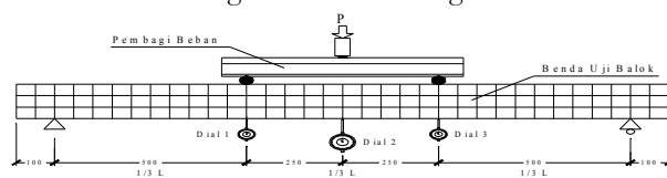
Gambar 5. Skema Pengujian Kuat Lentur
