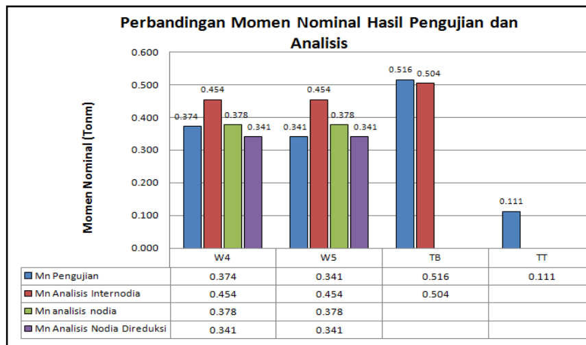
Gambar 7. Grafik Perbandingan Momen Nominal Hasil Pengujian dan Analisis
