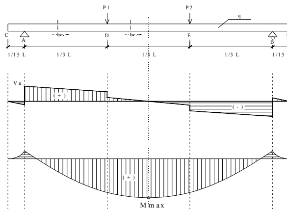
Gambar 2. SFD dan BMD
