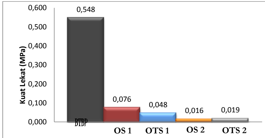
Gambar 3. Nilai Kuat Lekat Tulangan Baja Dan Tulangan Bambu Ori
