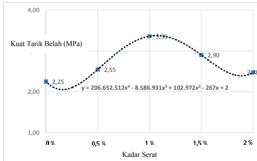
Gambar 2. Kurva regresi Hasil Pengujian Kuat Tarik Belah Beton
