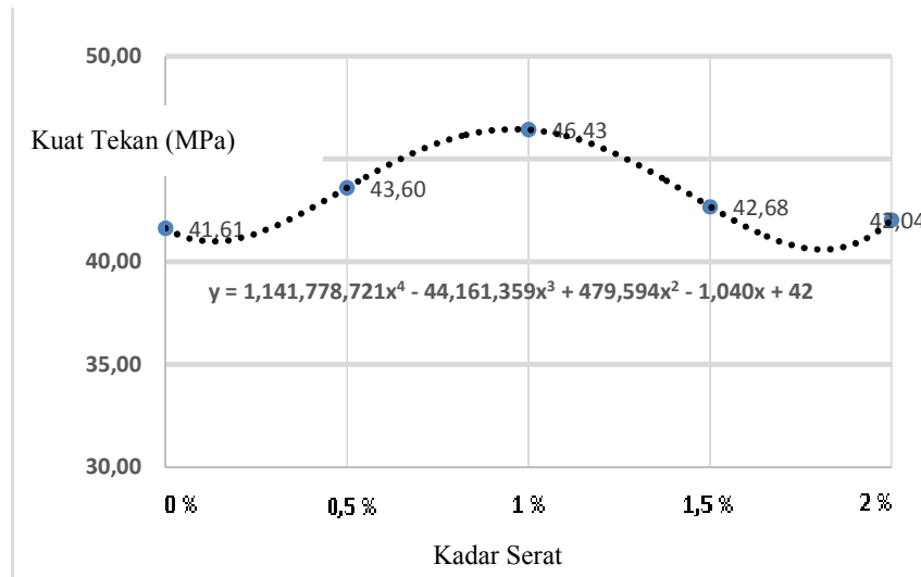
Gambar 1. Kurva regresi Hasil Pengujian Kuat Tekan Beton
