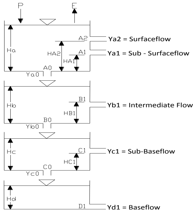
Gambar 2. Standar Tank Model untuk Analisis Keseimbangan Air Dinamis (Setiawan, 2003)
