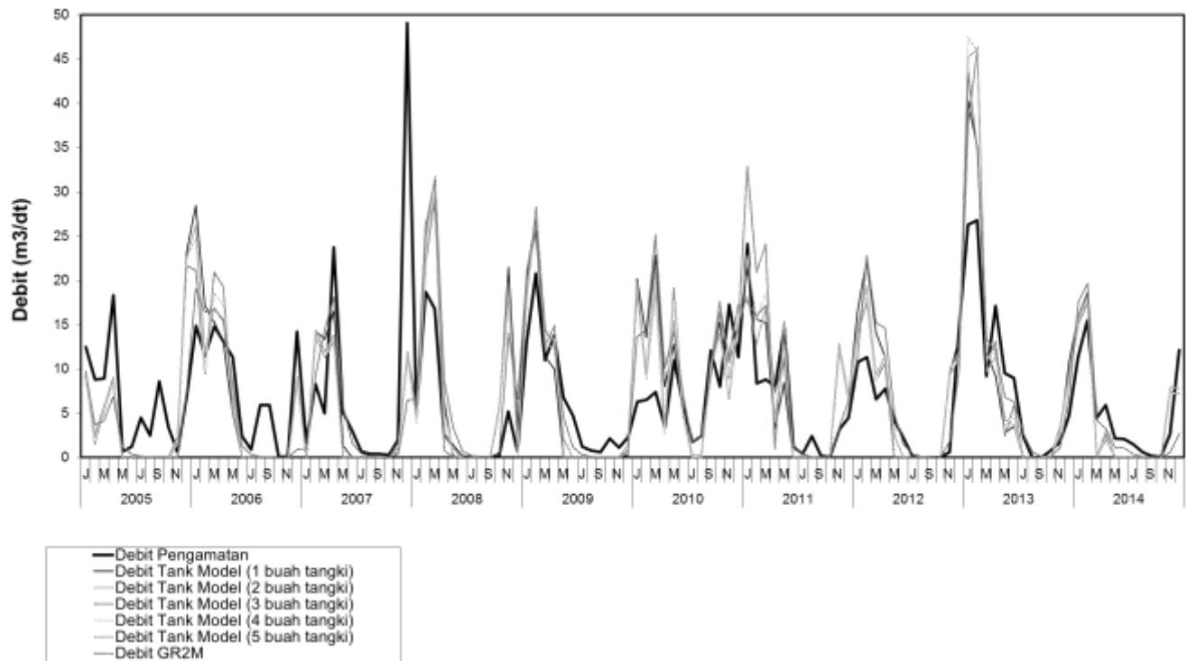
Gambar 4. Grafik Perbandingan Debit Transformasi dengan Debit Lapangan
