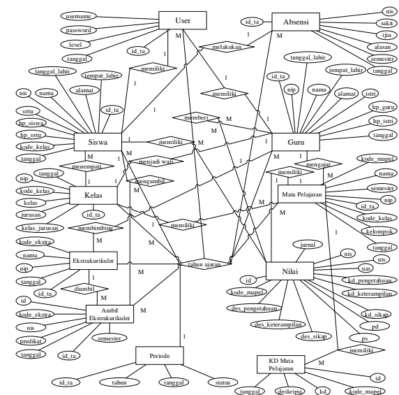
Gambar 9. Rancangan ERD
