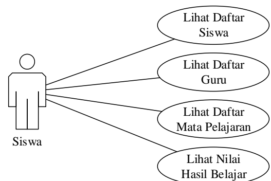
Gambar 3. Usecase Siswa
