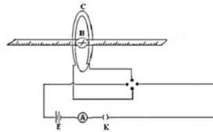
Gambar 7. Desain Alat Percobaan Induksi Magnet
