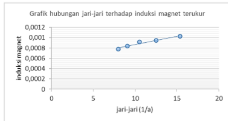
Gambar 9. Grafik Hubungan Jari-Jari Lingkaran (1/a) Terhadap Induksi Magnetik Terukur (B)
