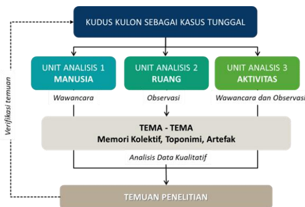
Gambar 1. Desain Penelitian
