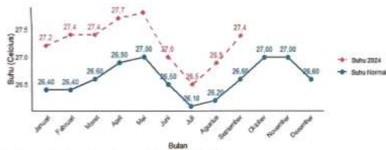
Sumber: Badan Meteorologi, Klimatologi, dan Geofisika, diolah Gambar 1.1 Suhu Normal Rata-Rata Bulanan Indonesia 1991-2020 dan Suhu Rata-rata Bulanan Indonesia Januari-September 2024
