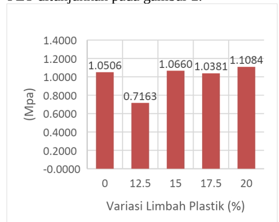
Gambar 2. Grafik kuat tekan bata ringan CLC umur 28 hari
