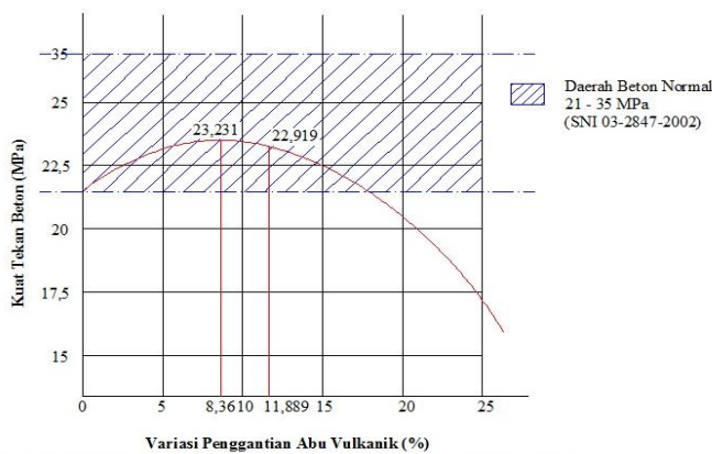
Gambar 6. Variasi Penggantian Abu Vulkanik Optimal pada Kuat Tekan Beton
