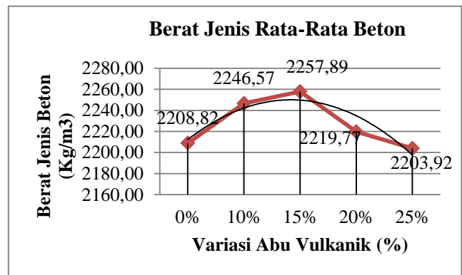
Gambar 5. Hubungan antara Persentase Abu Vulkanik dengan Berat Jenis Beton
