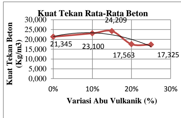
Gambar 4. Grafik Pengaruh Abu Vulkanik terhadap Kuat Tekan Beton
