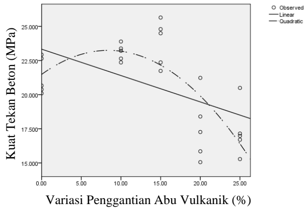
Gambar 3. Pengaruh Penggantian Abu Vulkanik Gunung Kelud terhadap Kuat Tekan Beton
