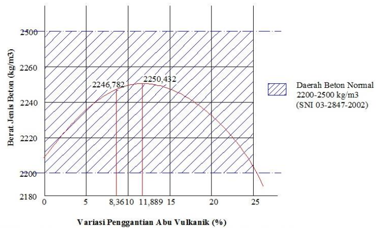
Gambar 7. Variasi Penggantian Abu Vulkanik Optimal pada Berat Jenis Beton
