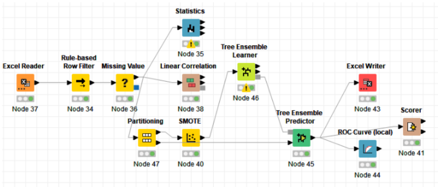
Gambar 3. Workflow Klasifikasi Tree Ensemble dengan SMOTE
