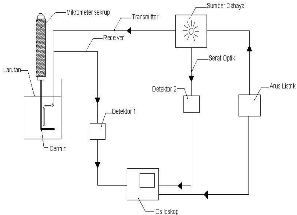
Gambar 1. Setup experimen fiber sensor untuk mengukur refraktif indeks larutan gula.
