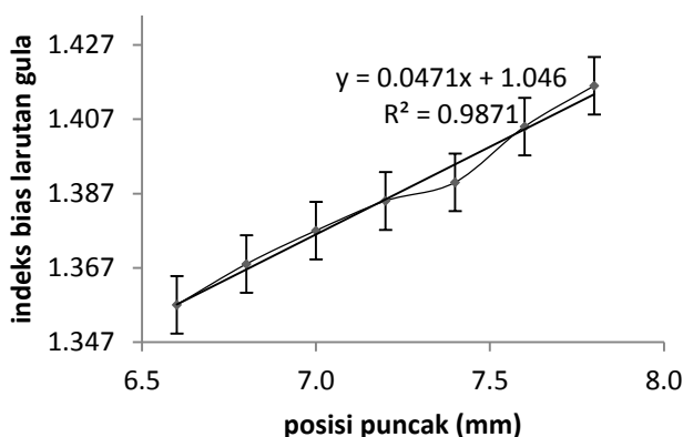
Gambar 4. Hubungan indeks bias dengan posisi puncak.
