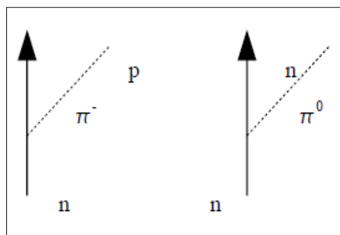
Gambar 1. Pemancaran Pion Virtual Oleh Nukleon [6].
