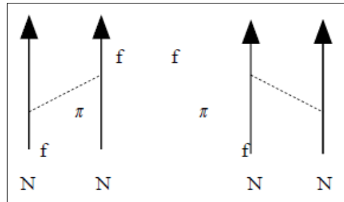
Gambar 2. Pertukaran Satu-Pion terhadap V_{NN} [6]
