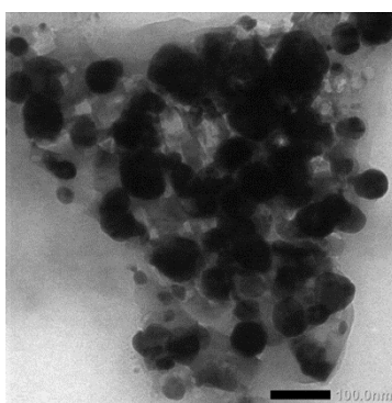
Gambar 7. Mikrograf TEM dari AgNPs.
