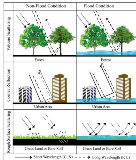
Gambar 2.2 Ilustrasi Mekanisme Backscatter Radar untuk Panjang Gelombang Pendek (C, X) dan Panjang (P, L) untuk kondisi banjir dan non banjir
