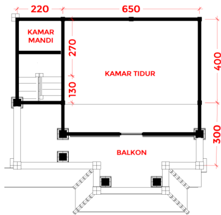
Gambar 6. Ukuran Zona C lantai 2 Sumber: Analisis Penulis, 2024
