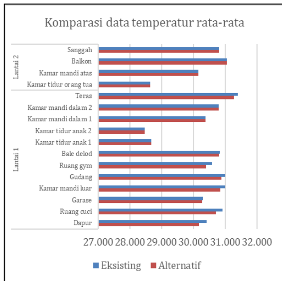
Gambar 13. Grafik Temperatur Rata-rata zona Sumber: Analisis Penulis, 2024
