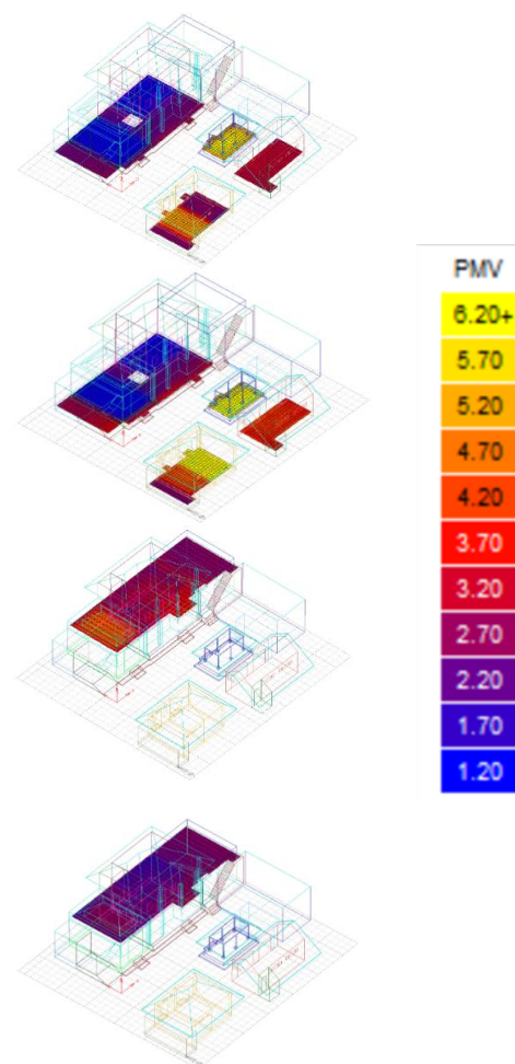
Gambar 10. PMV eksisting dan alternatif Sumber: Ecotect, 2024
