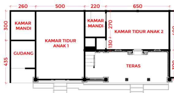
Gambar 5. Ukuran Zona C Sumber: Analisis Penulis, 2024
