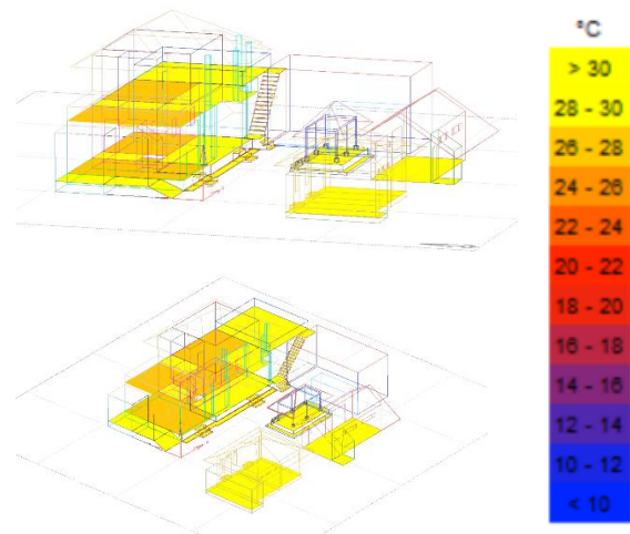
Gambar 8. Zone Temperature eksisting dan alternatif
