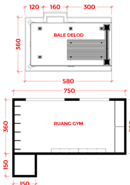
Gambar 4. Ukuran Zona B Sumber: Analisis Penulis, 2024
