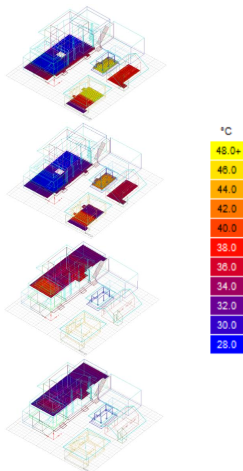
Gambar 9. MRT eksisting dan alternatif Sumber: Ecotect, 2024
