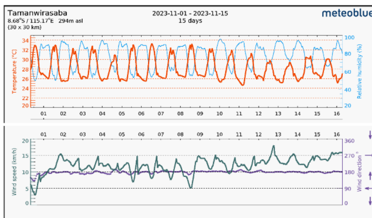
Gambar 7. Data cuaca 15 hari pertama Bulan November 2023 Sumber: meteoblue.com , 2024
