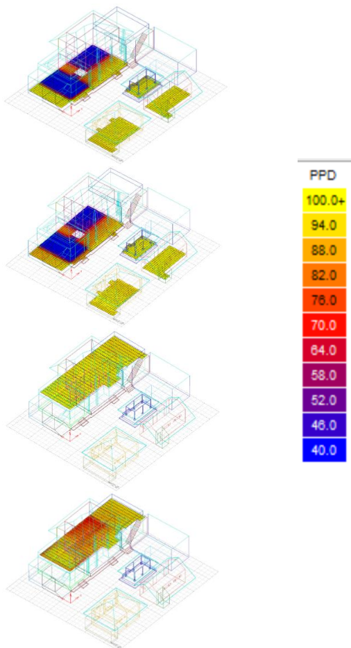
Gambar 11. PPD Eksisting dan Alternatif
