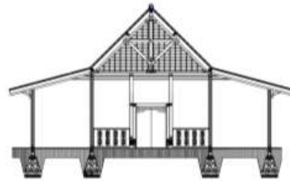
Gambar 12. Potongan Bangunan
